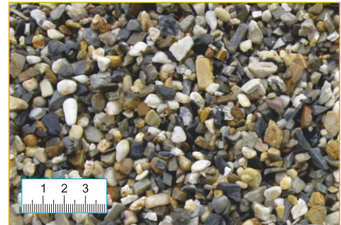
Fallschutzkies (Abb. 1:2,5)
