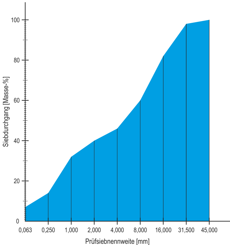
Schotterrasen gemäß FLL - Richtlinie
