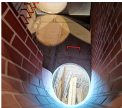
Schachtunterteile mit Rinne und Berme aus Kanalklinker
